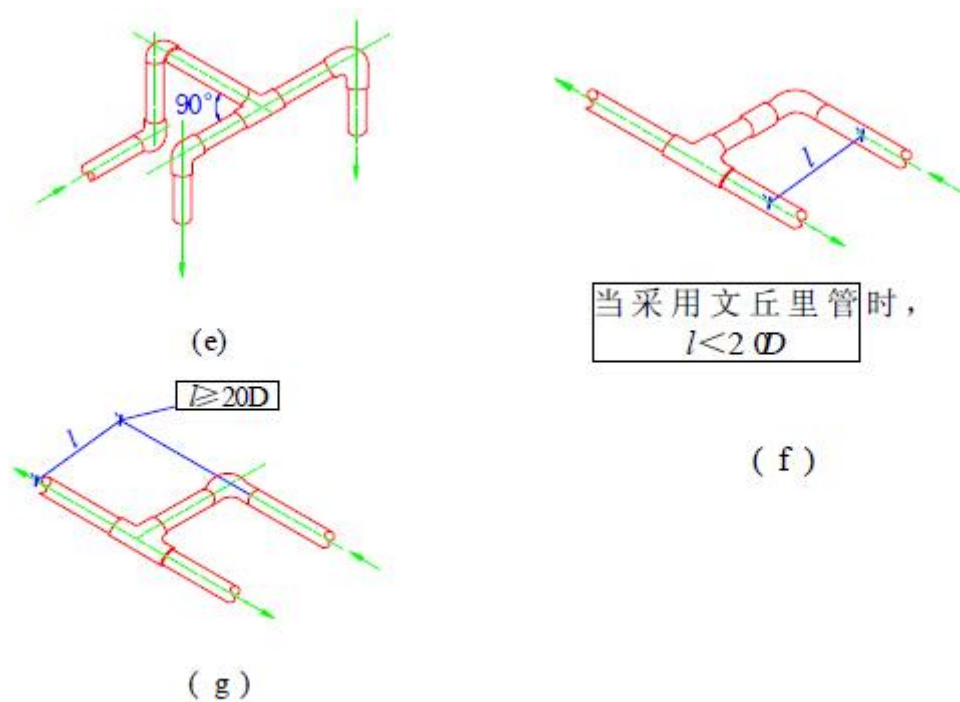
图 B 管网分支结构图
